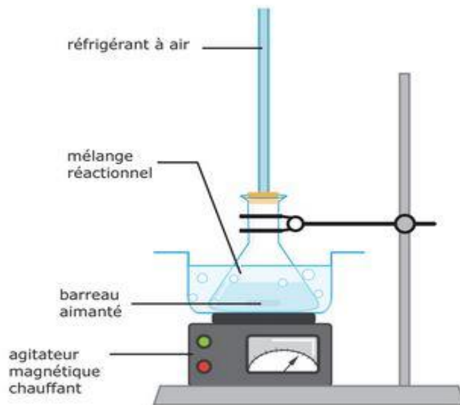
Chauffage à reflux avec réfrigérant à air
